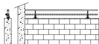
Appui Fenêtre + 1 tube
