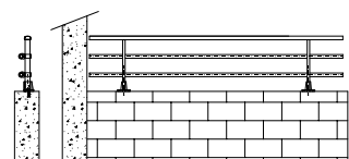
Appui Fenêtre + 2 tubes
